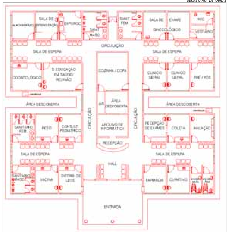
Planta Baixa: área construída de 626,82 m 2
