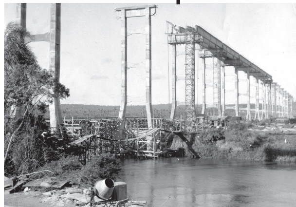
Ponte Carvalho Pinto em construção (1961).
